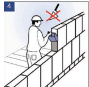
4 Empfehlenswert: Bei Pass- und Ergänzungselementen, Stoßfugen mit verleimen.
