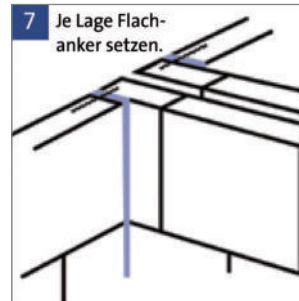
7 Anschluss Stabilitätswand mit tragen-de Wand, voll und satt verkleben.
