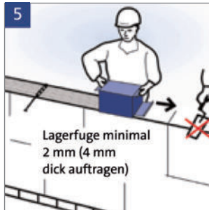
5 Lagerfuge minimal 2 mm (4 mm dick auftragen) Den Mörtelschlitten max. 2 Meter vor ziehen! Flacher Teil der Prik-Luftschichtanker mit geschlossener Seite oben, voll in das Mörtelbett legen.
