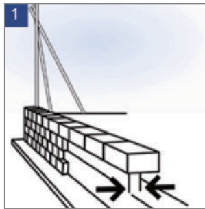
1 Kimmblöcke vollflächig unterfüttern. Zu kurze Decken sind zu verlängern. Stoßfugen der Kimmen vermörteln.
